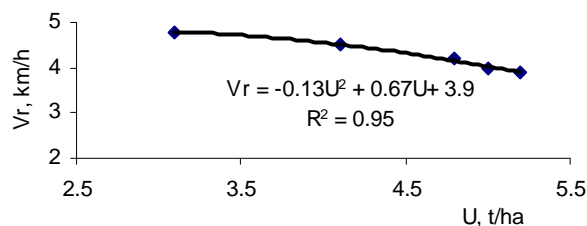
Figura 3. Velocidad de la cosechadora New Holland L-521.
