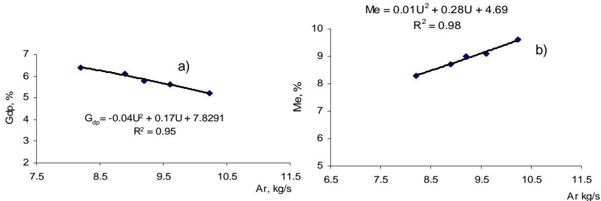
Figura 2. Comportamiento de la calidad del grano cosechado por la cosechadora New Holland L521 en función de la alimentación real. Grano pelado y quebrado ( G_{dp} ). ; b) Impurezas ( Me ).
