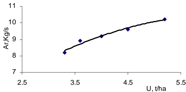
Figura 1. Alimentación real de la cosechadora New Holland L521 en función del rendimiento agrícola.
