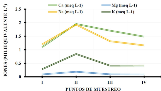
Figura 2. Comportamiento de los elementos Ca, Mg, Na y K en su transcurso por los puntos muestreados.
