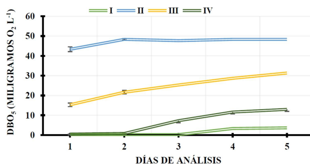
Figura 3. Evolución de la DBO 5 durante el período de análisis.
