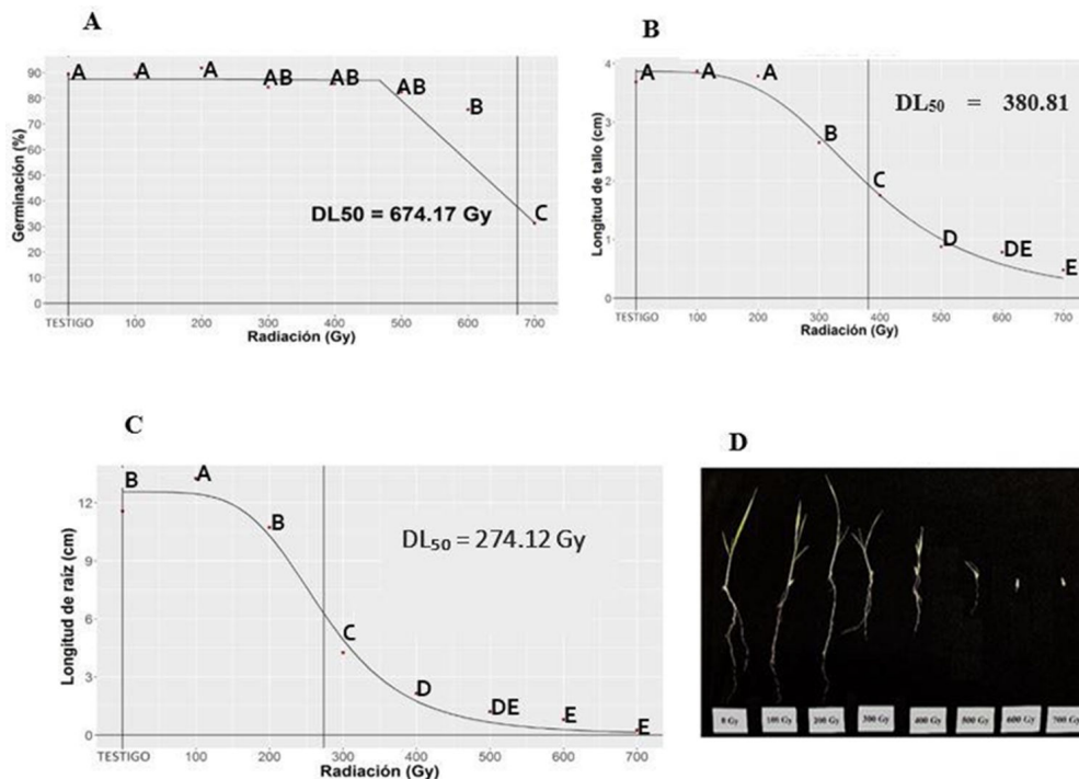
Figura 1. Irradiación con ^{60}\text{Co} en semillas de arroz ( Oryza sativa L. var CR5272) y su efecto sobre: el porcentaje de germinación (a); longitud del tallo (b); longitud de la raíz (c) y sensibilidad de CR5272 desde 0 hasta 700 Gy (d).
