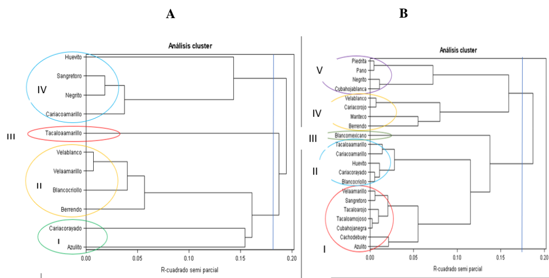
Figura 3. Dendrograma de 11 y 21 razas de maíz procedentes de los resguardos indígena del municipio de Tuchín Córdoba
