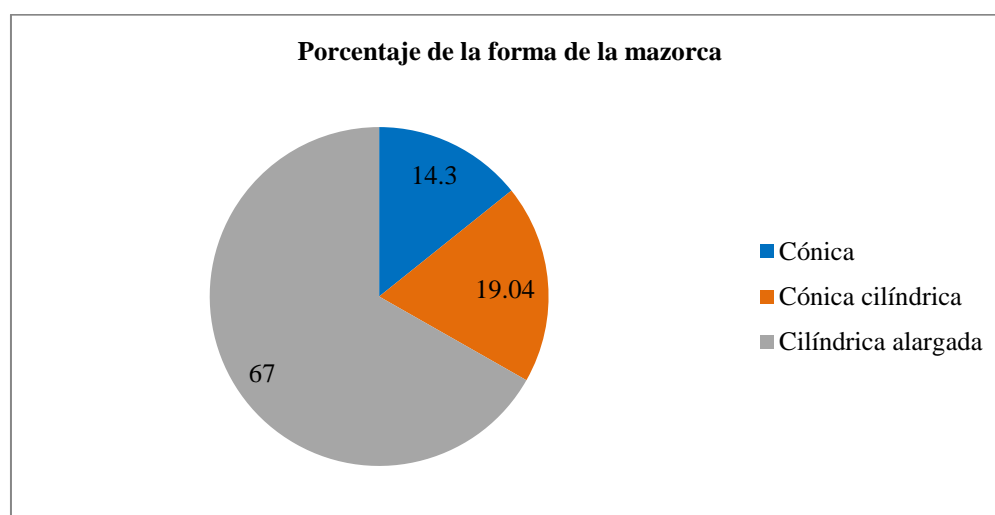
Figura 2. Porcentaje de forma de la mazorca
