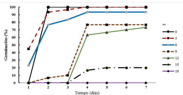
Figura 1. Efecto del polietilenglicol-6000 sobre el porcentaje de germinación de semillas de Phaseolus vulgaris L. cv. 'Delicias 364'.
