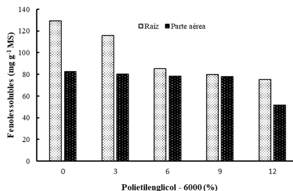
Figura 4. Contenido de polifenoles solubles en raíz y parte aérea de plántulas de Phaseolus vulgaris L. cv. 'Delicias 364' germinadas en condiciones de estrés hídrico
