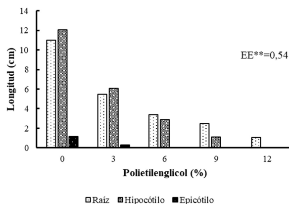
Figura 2. Efecto del PEG-6000 sobre el crecimiento de la raíz, el hipocótilo y el epicótilo de Phaseolus vulgaris L. 'Delicias 364'.
