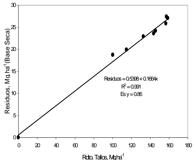
Figura 3. Modelación de la producción de residuos agrícolas cañeros en función del rendimiento de tallos en base húmeda cuando se realiza la cosecha sin la quema en Huixtla, Chiapas, Méjico
